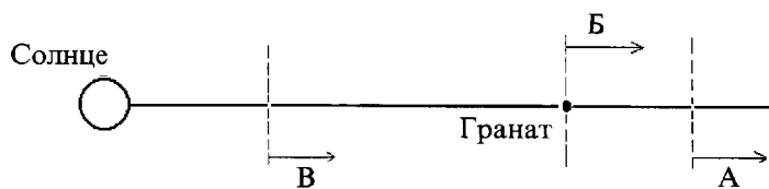
Рис. 2. Схема расположения передних фронтов возмущений от вспышек: А — фронт от вспышки F_1 , скорость фронта V = 685 км/с (или от F_2 , V = 1122 км/с); Б — от F_2 , V = 841 км/с (или от F_3 , V = 3461 км/с); В — от F_3 , V = 998 км/с (или квазистационарные неоднородности СВ и ММП от предыдущих вспышек)
