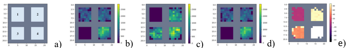
Рис.3. Экспериментальные результаты: (a) схематичное изображение объекта; (b,c,d) экспериментально измеренные кросс-корреляционные функции G^{xy}(r) , G^{yx}(r) и G^{TA}(r) , соответственно. Шкалы даны в пикселях, полный масштаб 930 \mu\text{m} ; e) поляризационное фантомное изображение \theta(r) 4-х секционного образца.
