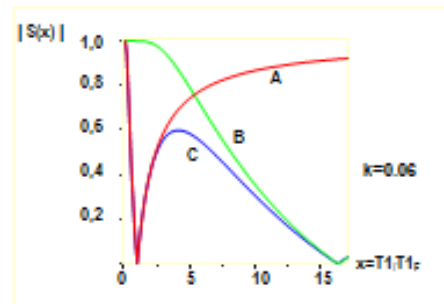
Рис. 2. Зависимость МР сигнала от времени T1 для разных методов сканирования: А - STIR, В - FLAIR, С – двойная инверсия-восстановление.
