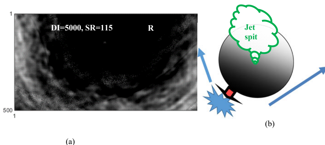
Рис. 2. В R канале SR изображения (а) видим сдавливаемый кластер звезд и две трубки звездотоков, см схему (b), направление Jet spit - вверх см. Рис. 1 (b) по G каналу.
