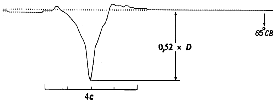
Рис. 35. Форма импульса смещения в ближней зоне для землетрясения типа правостороннего сдвига и скорости вспарывания, равной 2,2 \text{ км/с}
